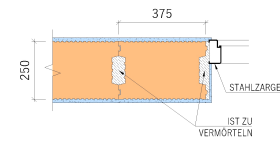
- VERBUND AN DER TÜRLAIBUNG, 1. REIHE DES MAUERWERKS
