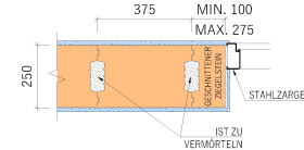
- VERBUND AN DER TÜRLAIBUNG, 2. REIHE DES MAUERWERKS
